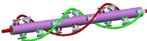
Rotor sa duplospiralnom raspodjelom
